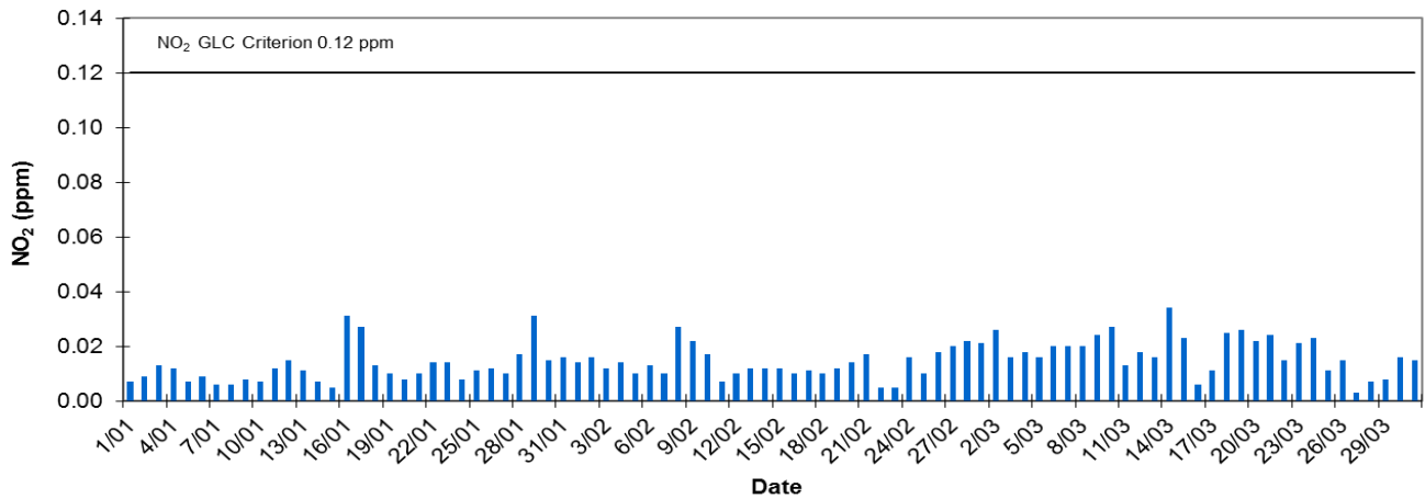
Le Fevre 2 1 Hr Daily Maxima NO2 - Quarter 1, 2017
