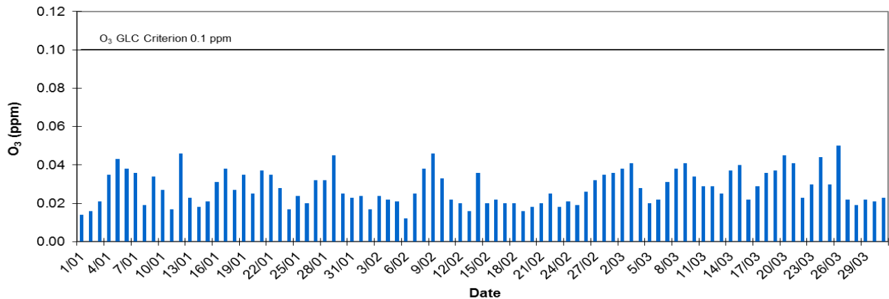
Le Fevre 2 1 Hr Daily Maxima O3 - Quarter 1, 2017
